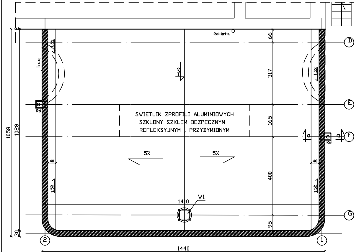
RZUT DACHU 1:100
