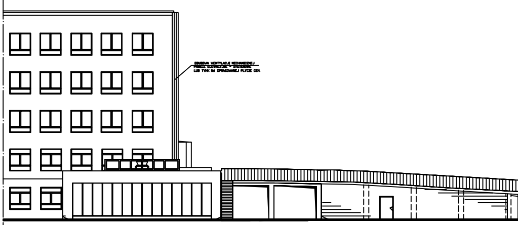
ELEWACJA POŁNOCDNA PROJEKTOWANY PODJAZD KARETEK POCHYLNIA POMIESZCZENIA TECHNICZNE
